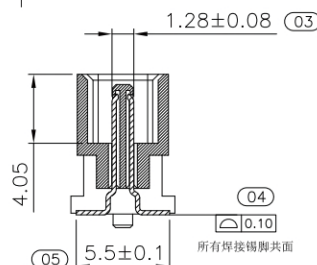
剖面 A-A
